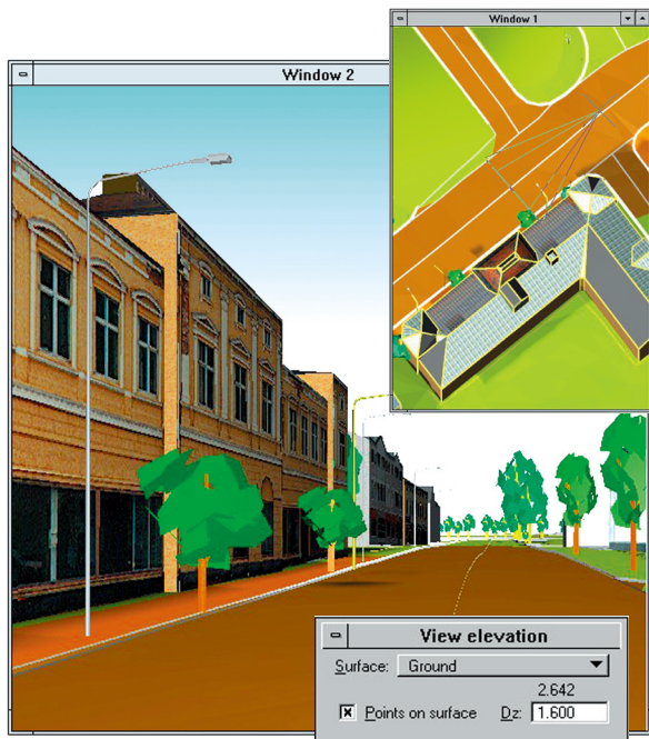
TerraModelerは、サーフェス・モデルの高さに則して、要素を正しい高さで対話的に配置することが出来ます。
